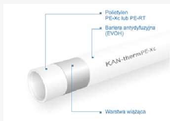
rury jednorodne
